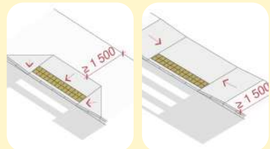
Приклад влаштування бордюрного пандусу (розміри вказані у мм)
